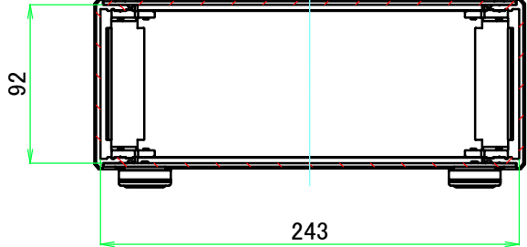
A-A ( 1 : 4 )
